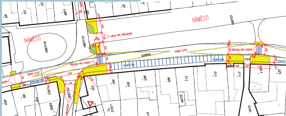
Schválený návrh řešení přechodů v Proseči
